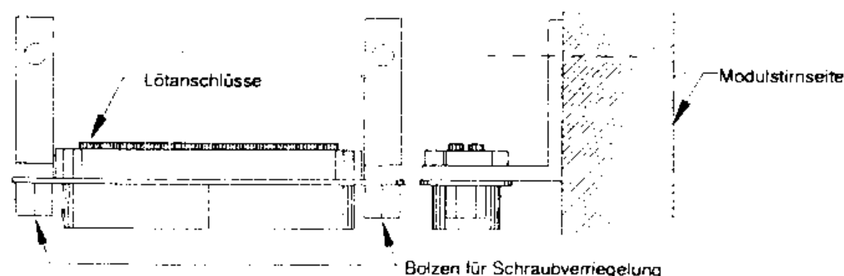
Abb. 1 Empfehlung für die Montage der Stiftleisten im Modul (Detail)
