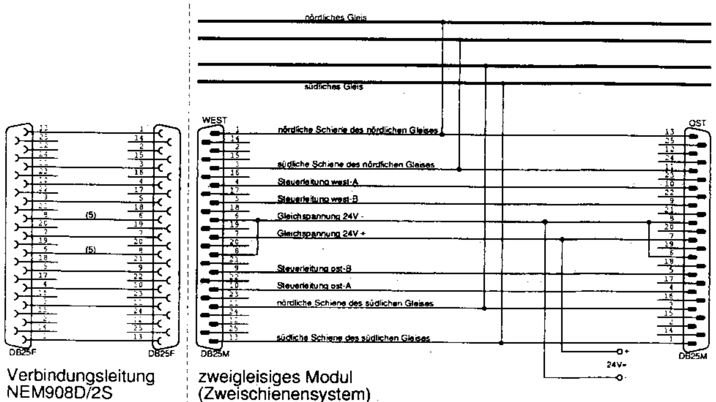
Abb. 4 Verdrahtung bei zweigleisigem Modul nach dem Zweischienensystem / Verbindungskabel hierzu
