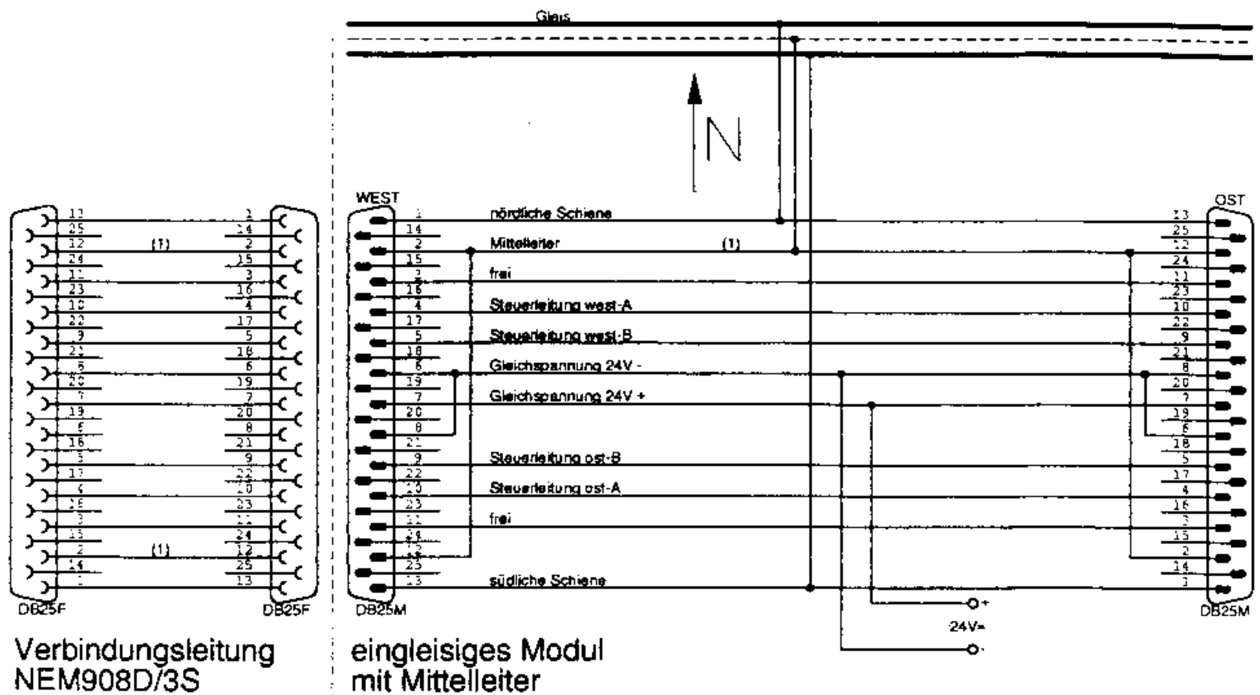
Abb. 3 Verdrahtung bei eingleisigem Modul mit Mittelleiter / Verbindungskabel hierzu
