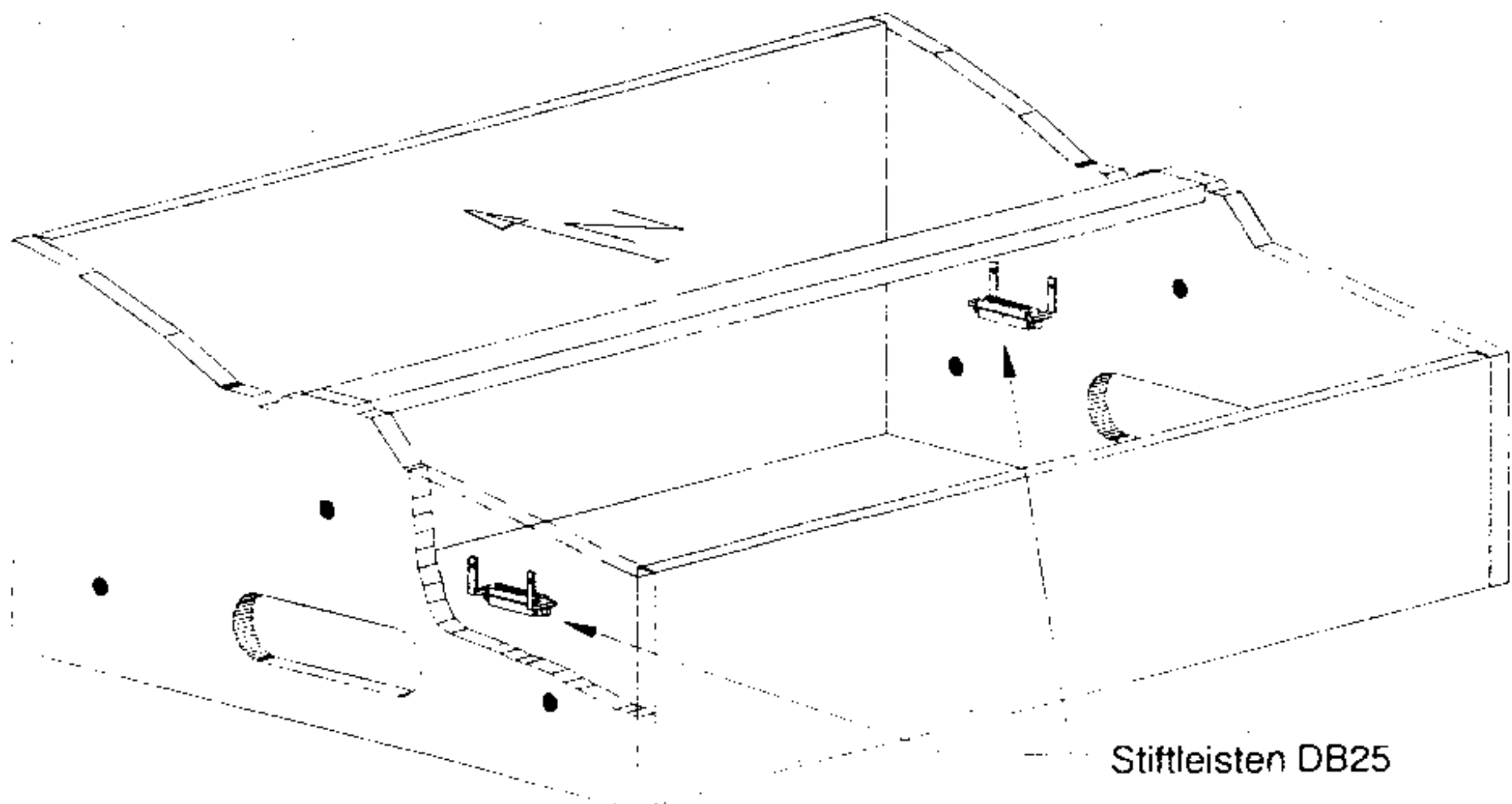
Abb. 2 Empfehlung für die Montage der Stiftleisten im Modul
